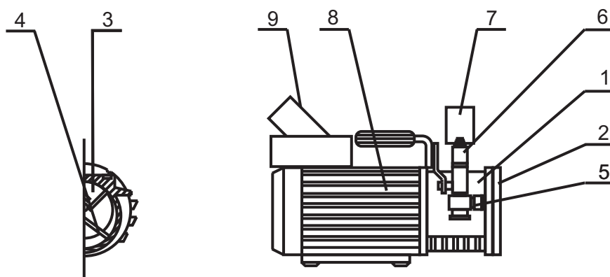
Budowa agregatu zasysającego AZ-15.
